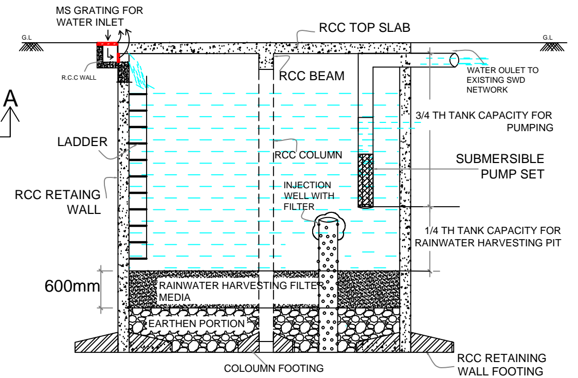
SECTION A-A
